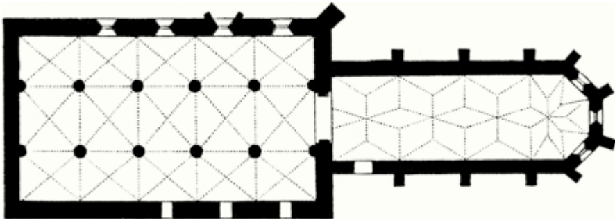
Abb. 216: Grundriss der Dominikanerkirche in Retz
