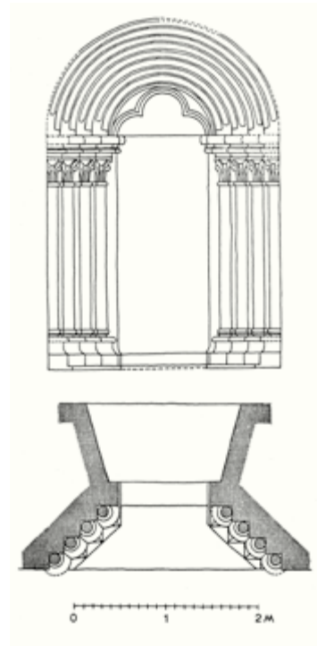
Abb. 196 a und b: Südportal der Stiftskirche in Kremsmünster, Ansicht und Plandarstellung
