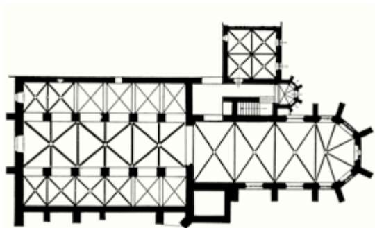
Abb. 183: Grundriss der ehem. Minoritenkirche in Stein
