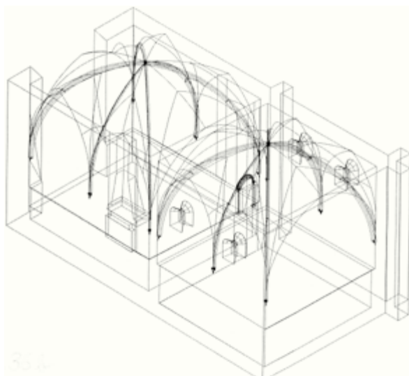
Abb. 36 a und b: Babenbergerpfalz in Klosterneuburg. Baureste des Palas und Rekonstruktionszeichnung
