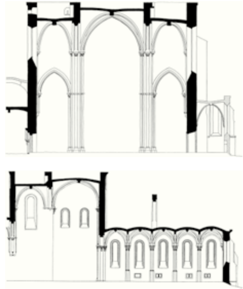
Abb. 29: Aufrisschnitt durch das östlichste Langhausjoch der Stiftskirche Lilienfeld
