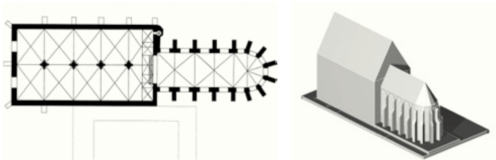
Abb. 191 a und b: Rekonstruktion des ersten Bauzustandes der Minoritenkirche in Wien, Grundriss und Baumassenmodell
