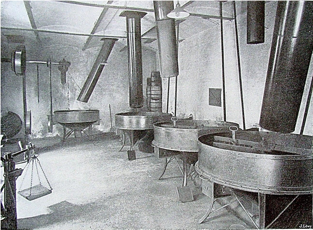
Der Kühlraum für die gebrannten Kaffees.
