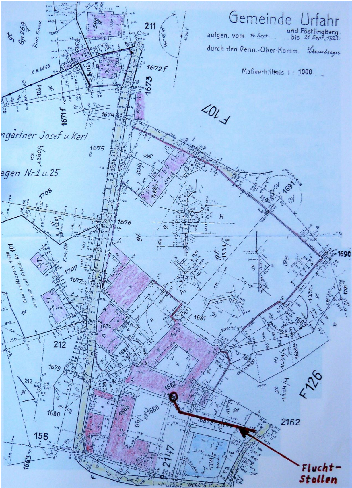
Lageplan des am 28. Juli 2011 entdeckten Fluchtstollens des ehem. Schlosses Hagen (Vermessung D.I. Lipp) (Darstellungs-Grundlage: Plan der Gemeinde Pöstlingberg vom 21. September 1921; ASTL)
