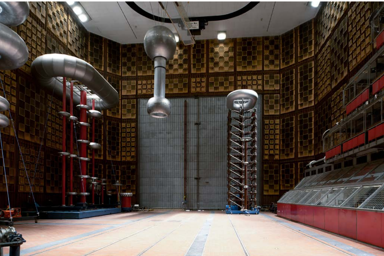
Abb.: Hochspannungshalle – Innenansicht (Foto: H. Tezak)
