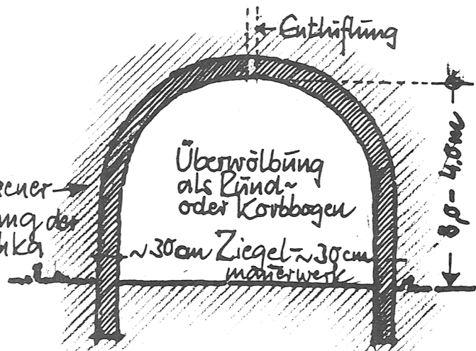
Querschnitt a ~ a
